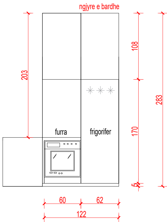
PAMJE 3-3
