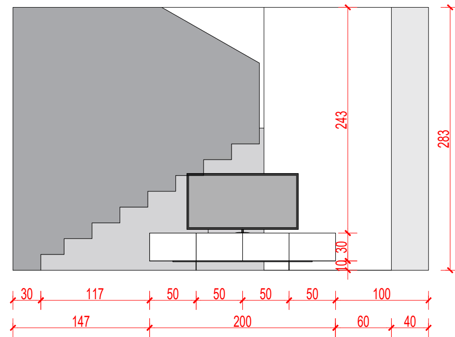
PAMJE 1-1
