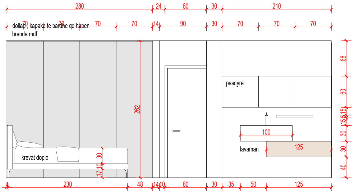
PAMJE 3-3
