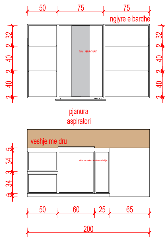
PAMJE 2-2
