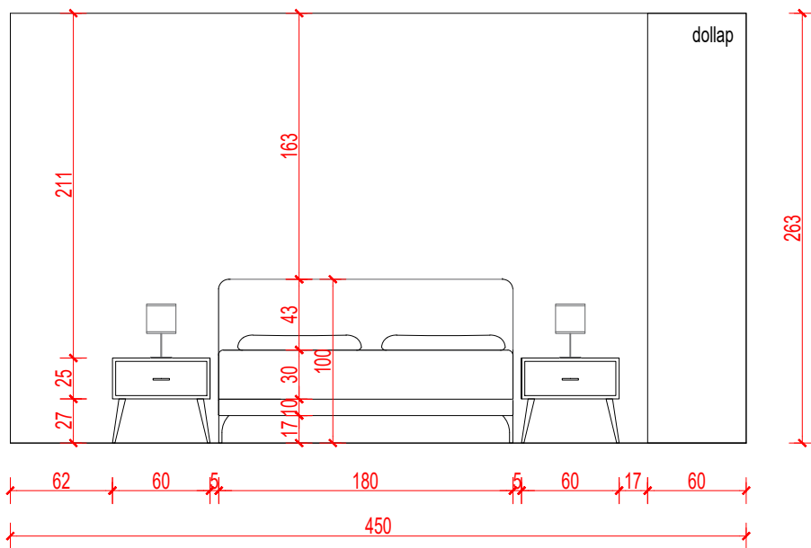
PAMJE 1-1
