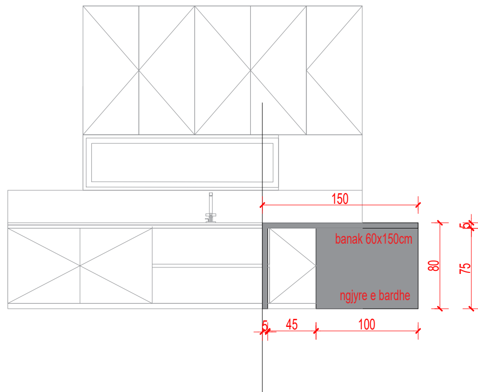
PAMJE 4-4
