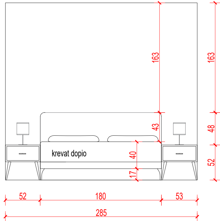
PAMJE 2-2
