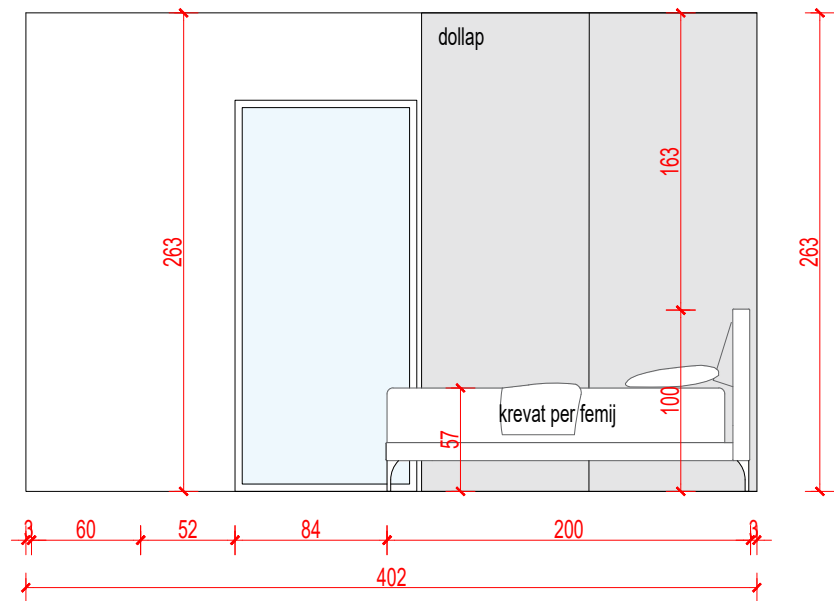
PAMJE 3-3
