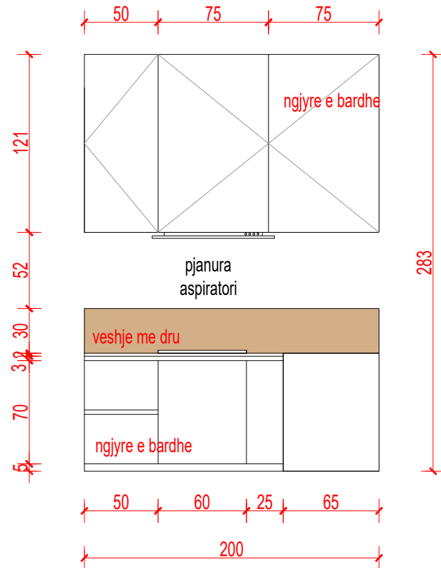
PAMJE 2-2
