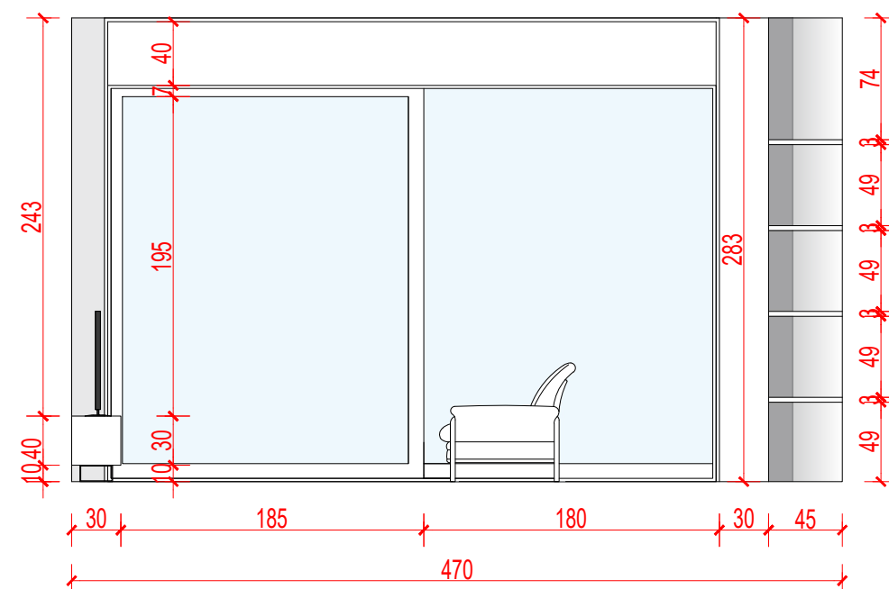
PAMJE 2-2
