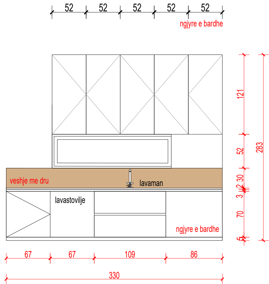
PAMJE 1-1
