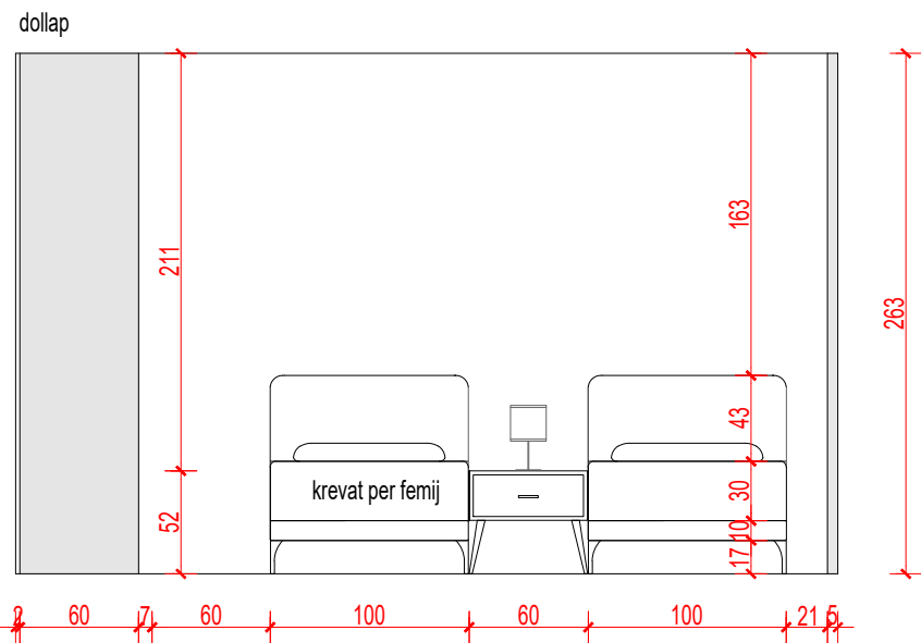
PAMJE 1-1
