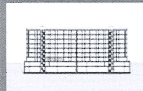
SEKSIONI C
